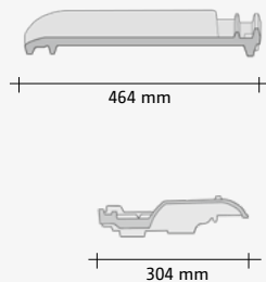
Entlüfter/Ton-Solar-Abdeckziegel Ventilatiepan/Klei solar montagepan Chatière/ Tuiles pour couvrir les crochets de montage solaire
