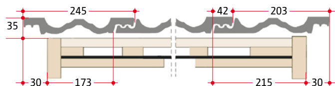
Maße Doppelkremper
