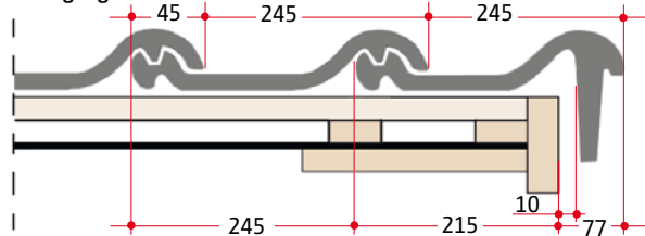
Maße Doppelkrempen
