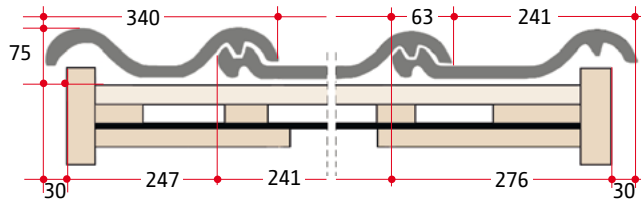
Maße Doppelkremper
